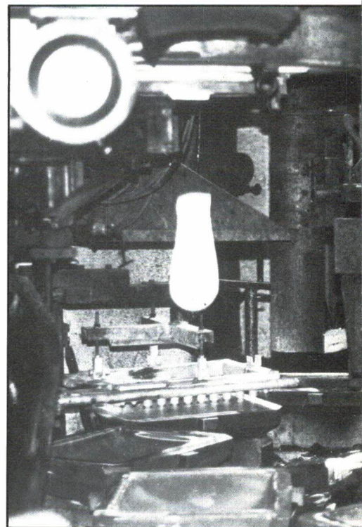
Geboorte van de beeldbuisconus. Zwaar valt de enorme, gloeiende glasdruppel in de persvorm.
