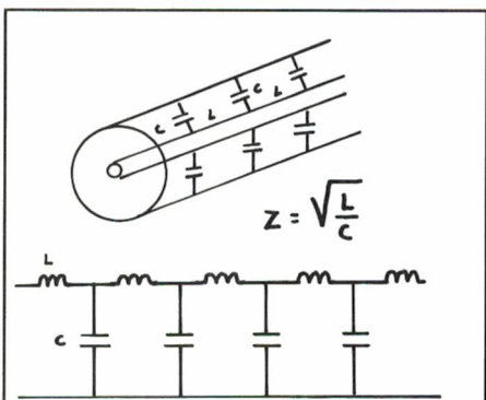
Fig. 4. Een coaxkabel heeft zelfinductie (L) en capaciteit (C). De wortel uit de L/C verhouding bepaalt de karakteristieke impedantie.
